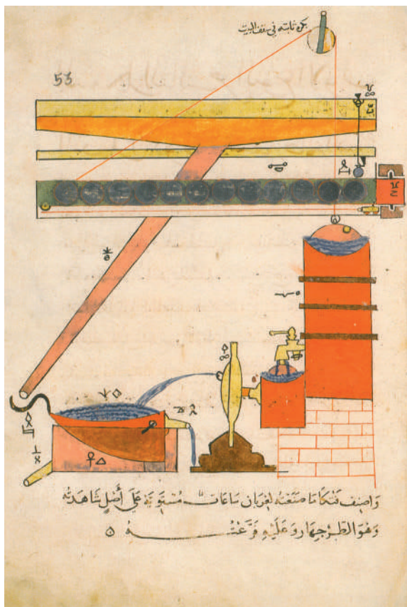
Рис. 18.14. Одна з механічних конструкцій Аль-Джазарі.
